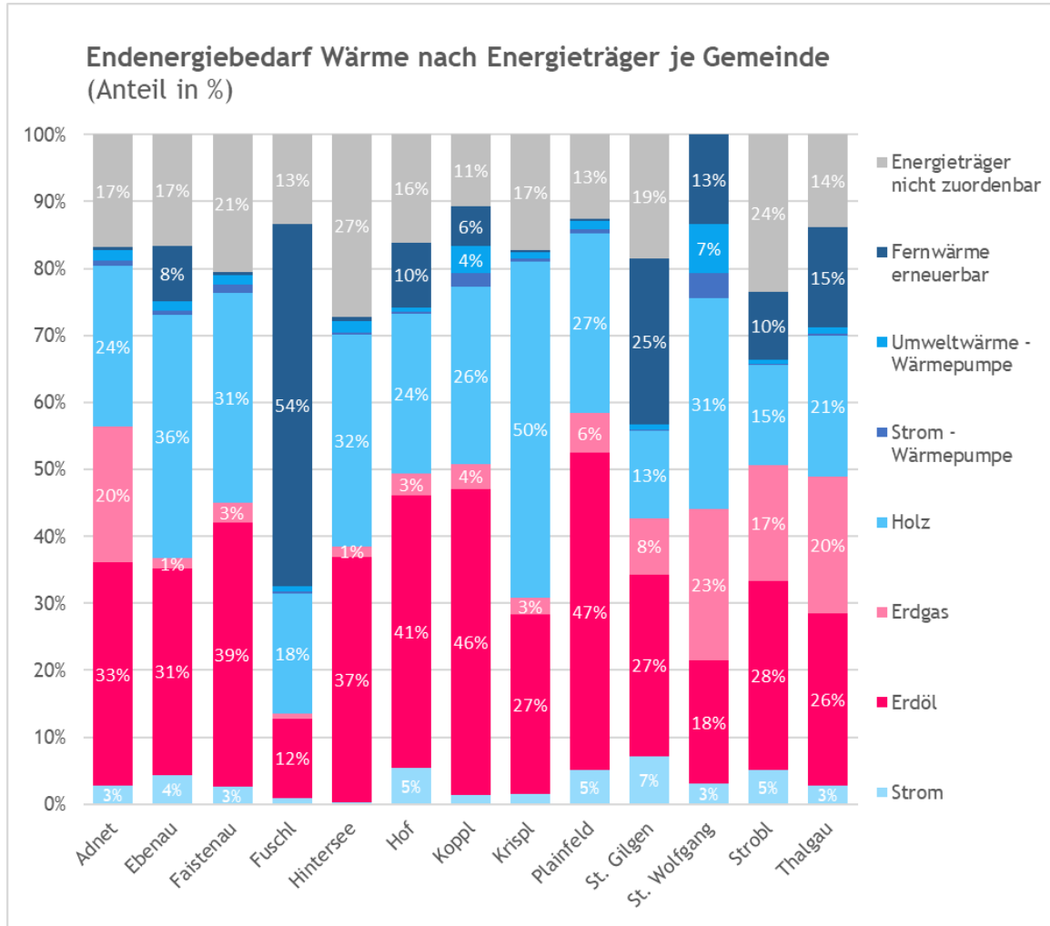
Abbildung 22: Modellierter Wärmebedarf nach Energieträger je Gemeinde (Daten: Bestandsanalysen Energie Salzburg, Emissionskataster OÖ) (Quelle: Standl et al., 2022)
