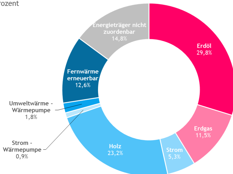
Abbildung 21: Energiebedarf Wärme nach Energieträger in den Gemeinden der KEM Fuschlsee - Wolfgangsee 2021 (Quelle: Standl et al., 2022)
